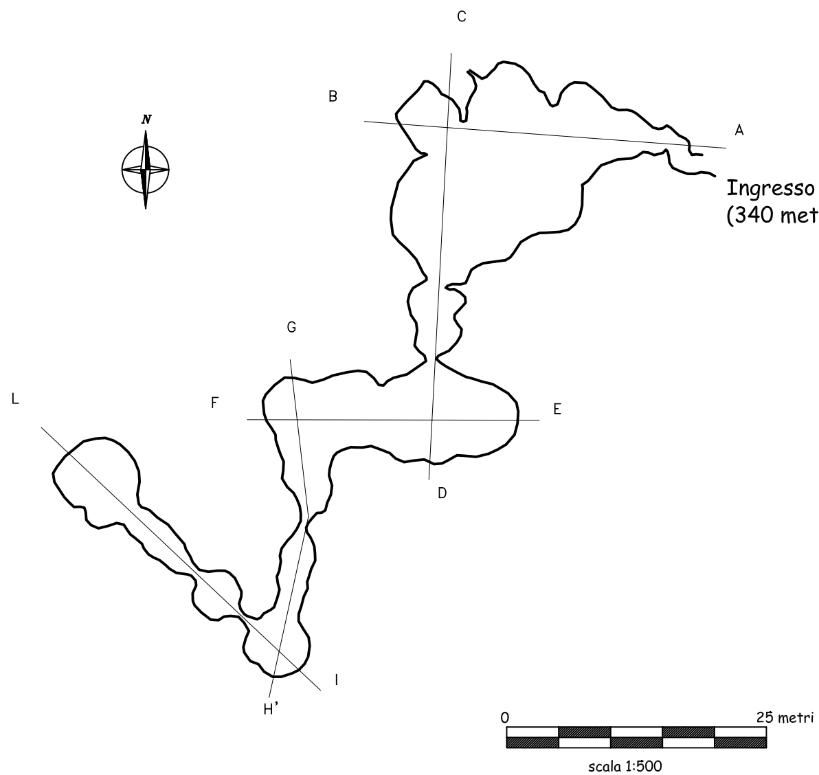
Pianta 1:500
