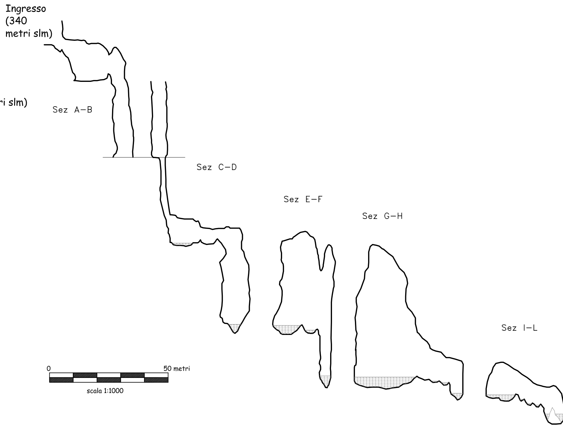
Sezione longitudinale 1:1000
